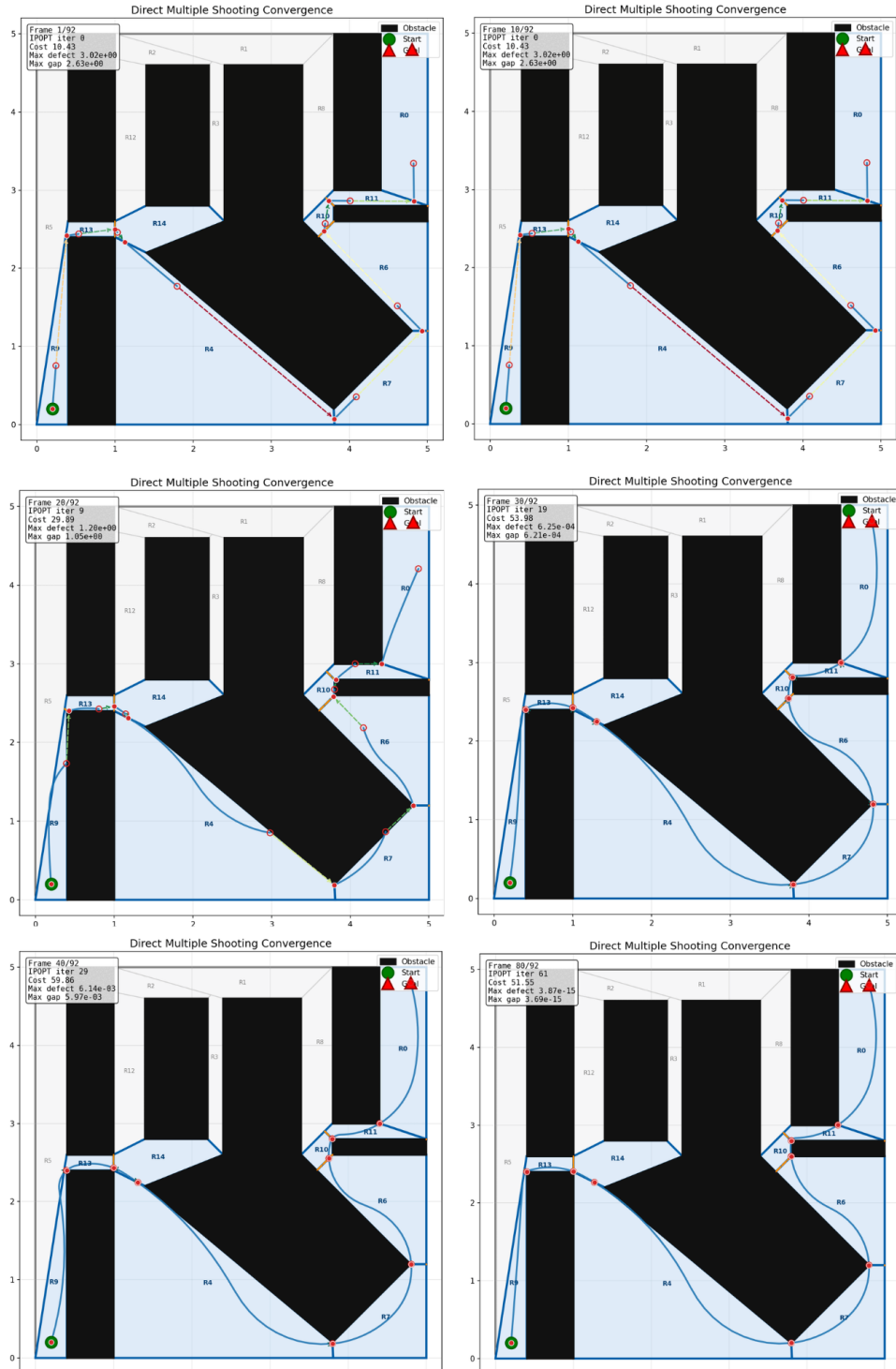
Hình 5.4: Quá trình hội tụ của GCS-DMS trên môi trường 2D đơn giản. Các khung hình thể hiện sự giảm dần của defect dynamics và connection gap trong quá trình tối ưu.
