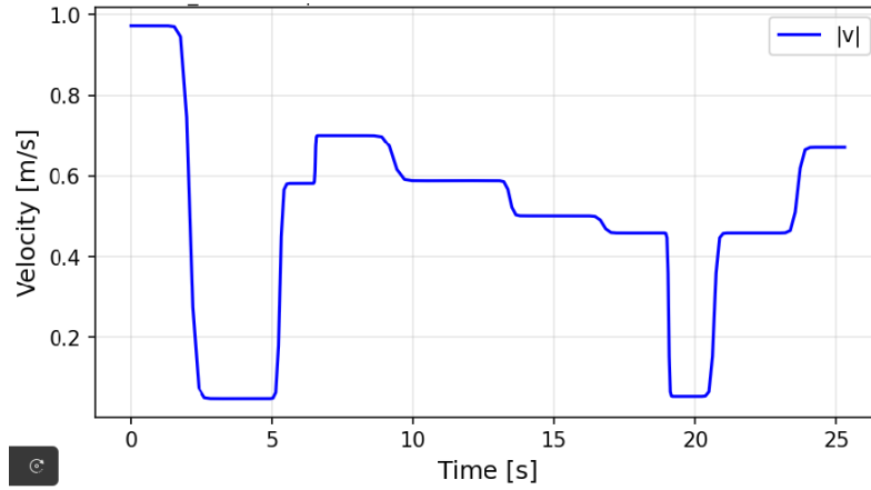
Hình 5.5: Hồ sơ vận tốc của nghiệm GCS-DMS trên môi trường 2D đơn giản. Vận tốc giảm tại các đoạn cua và tăng trở lại ở các đoạn có hình học thuận lợi hơn.
